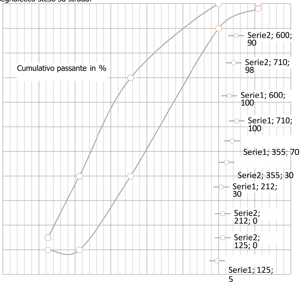
Grafico 1 – Fuso granulometrico di riferimento delle microsfere di vetro da postspruzzare costruito sulla base Luce netta in micron dei setacci ISO 565 – R 40/3 dell'esempio 2 (600-125 micron) – prospetto 4 della UNI EN 1423 – Tabella 14 del Capitolato
