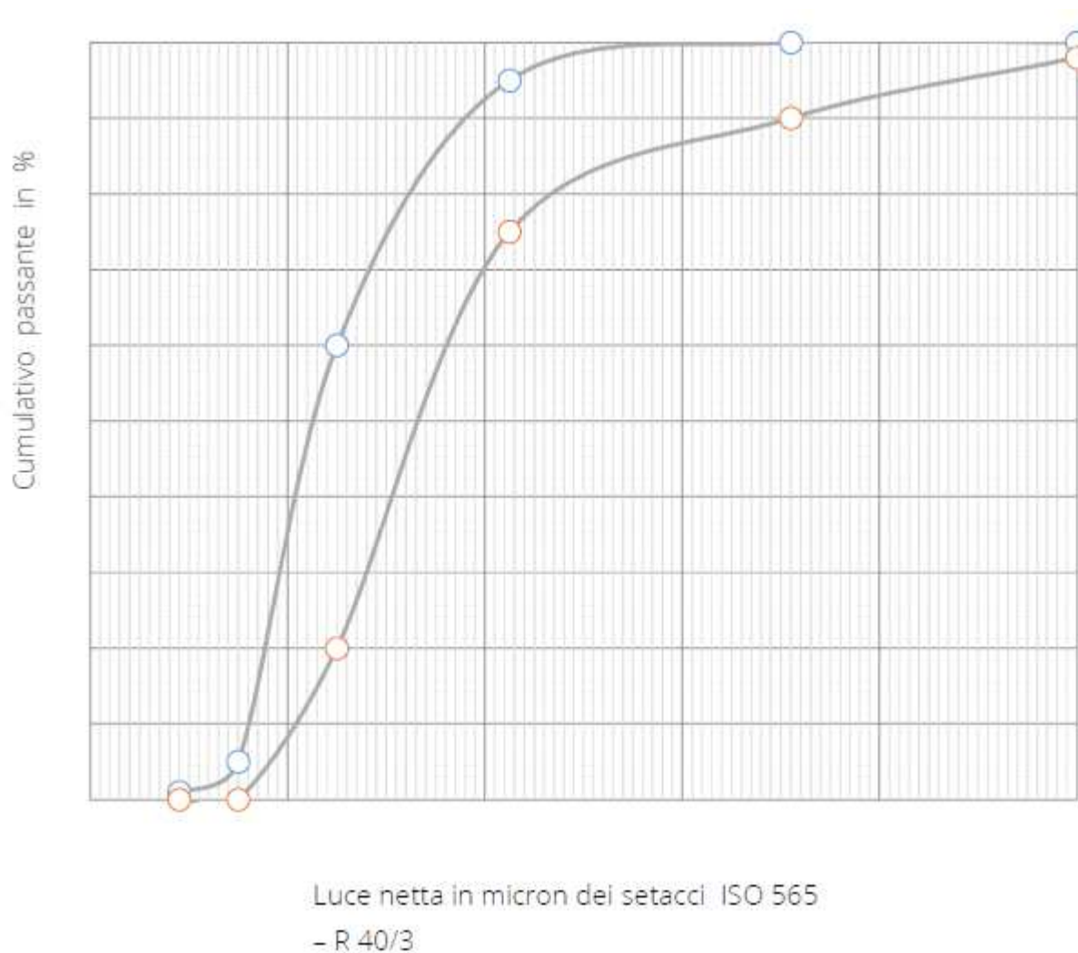
Grafico 2 – Fuso granulometrico di riferimento dei granuli antiderapanti da postspruzzare, trasparenti e non trasparenti, costruito sulla base degli esempi 3 e 5 (710 -150 micron) – prospetto 10 della UNI EN 1423 – Tabella 16 del Capitolato
